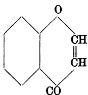
Chromon
